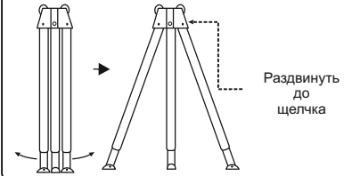
Рис. 3. Фиксация опор
