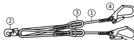
СТРОП ДВОЙНОЙ УДЕРЖИВАЮЩИЙ KNT05F, KNT22
