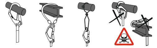
Рис. 9. Использование стропов без амортизатора
