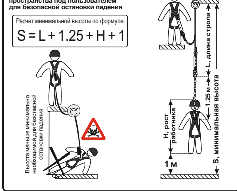
Рис. 10. Расчет высоты свободного пространства под пользователем для безопасной остановки падения
