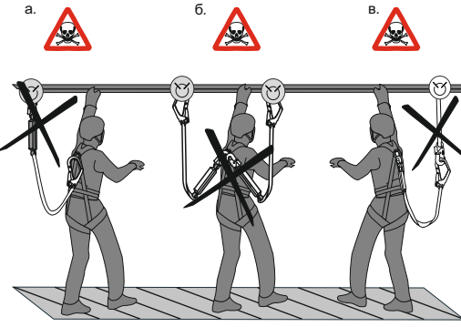
Рис. 11. Ограничения по использованию стропов с амортизатором
