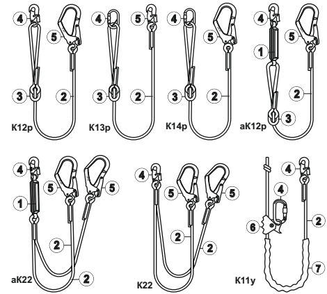
Рис. 1. Внешний вид, состав стропов
