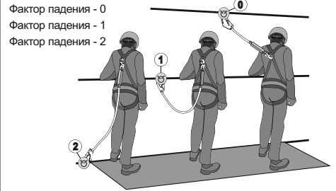
Рис. 5. Использование стропа с амортизатором рывка
