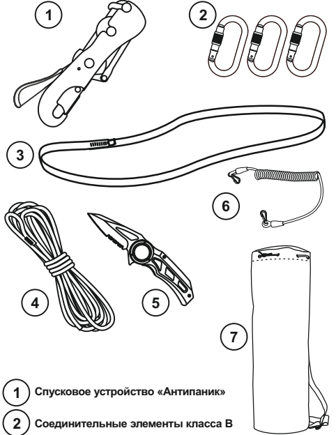
Рис. 1. Состав комплекта
